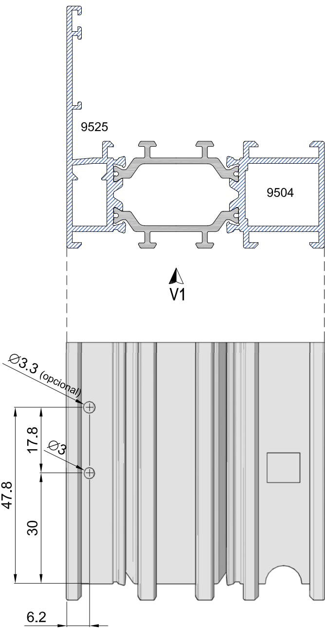
Mecanizado escuadra exterior V1 M3 1:1
