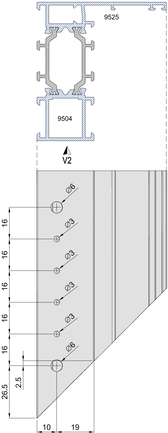
Mecanizado bisagra WINKHAUS M8
