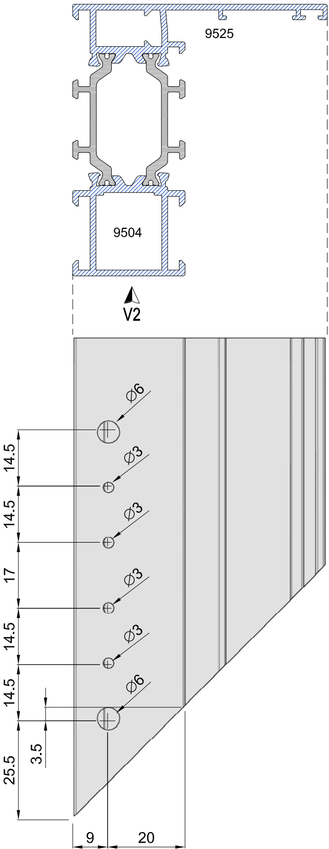
Mecanizado bisagra VBH M9 (posición intercambiable)
