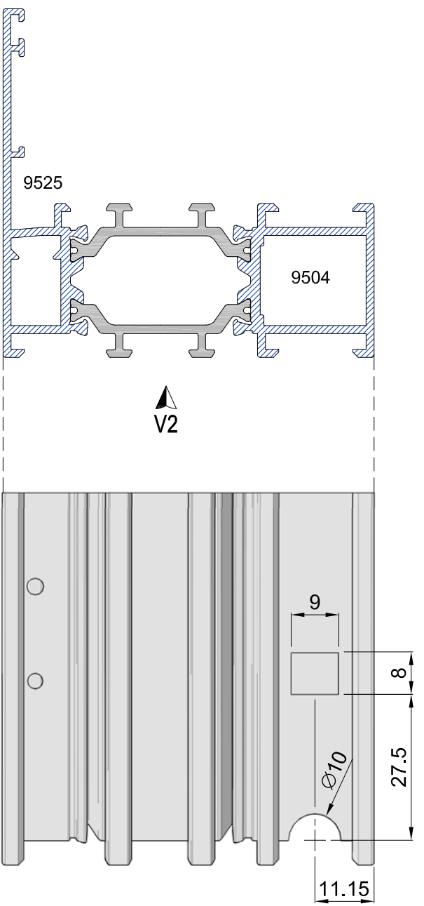
Mecanizado escuadras familia 26 V2 M7 1:1
