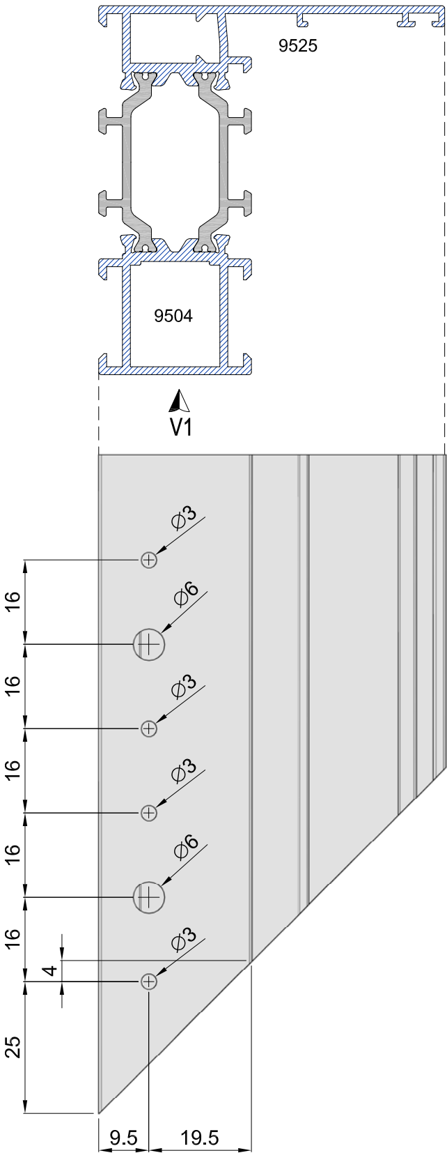
Mecanizado bisagra ROTO M9 (posición intercambiable)
