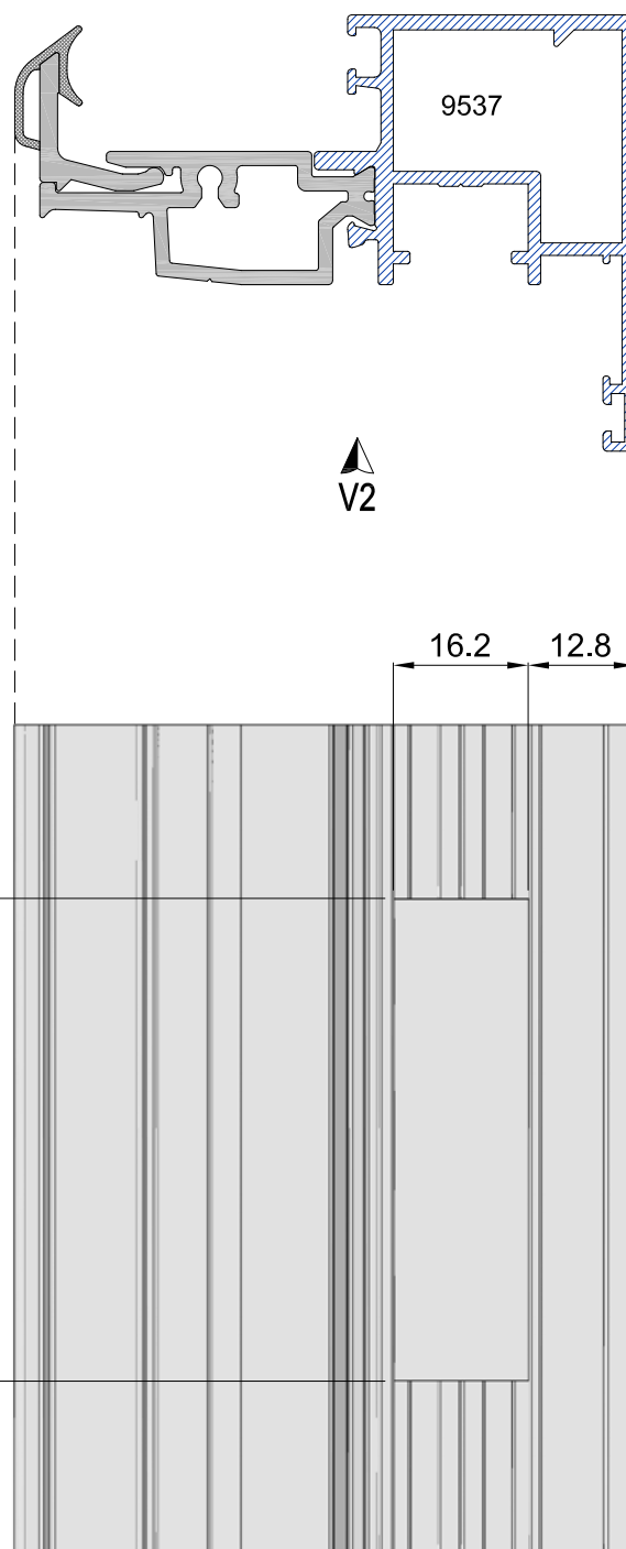
Mecanizado caja cremona M6
